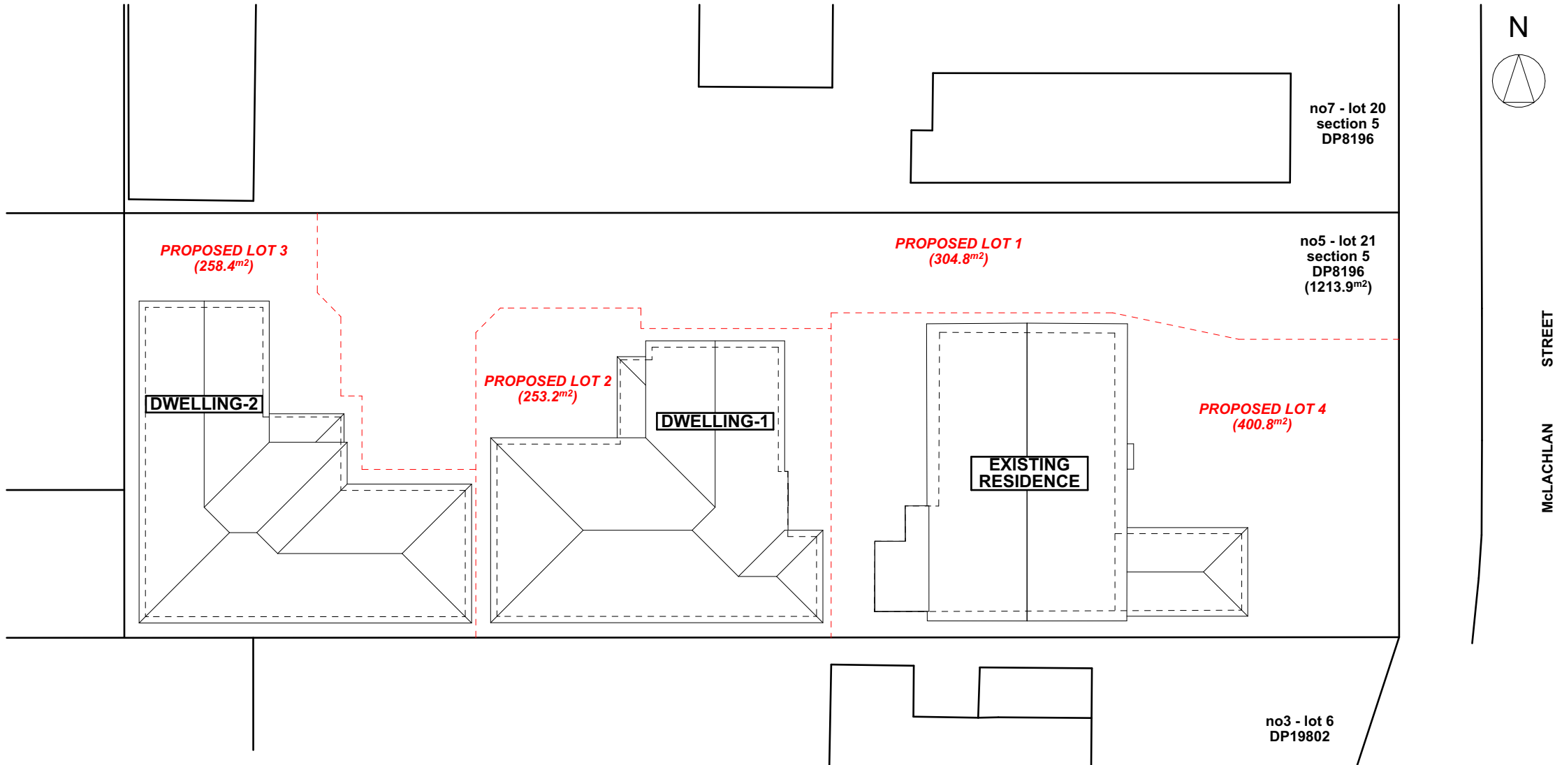
SUBDIVISION PLAN 1:250
