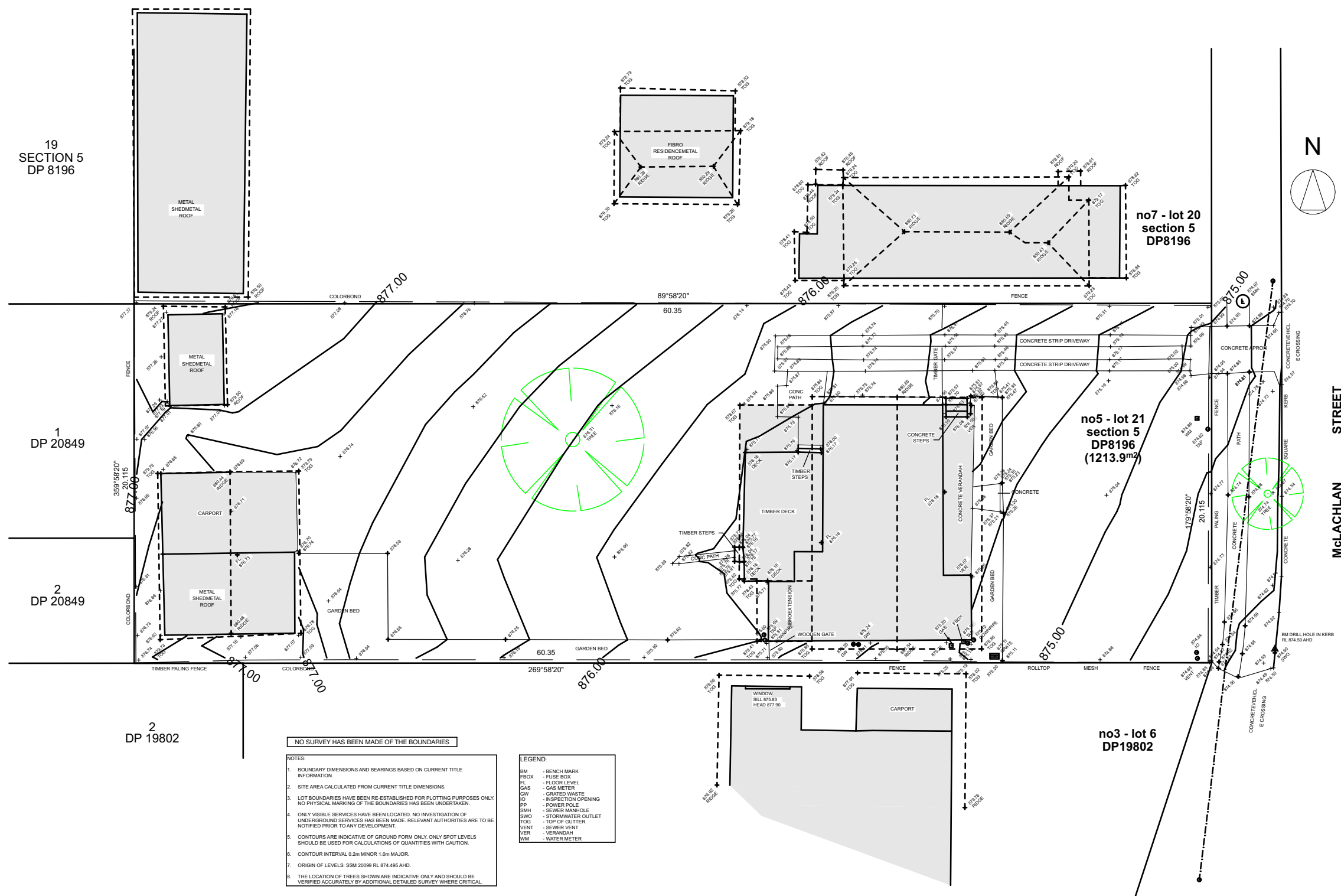
EXISTING SITE PLAN 1:250
